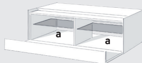
CO3
