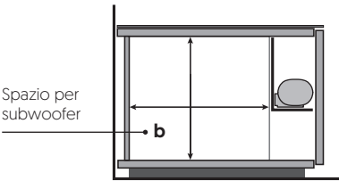
b = Dimensioni dietro soundbar
